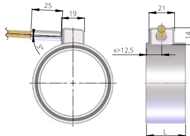
Abb. 11: Düsenkappe tangential fig. 11: tangential nozzle cap
